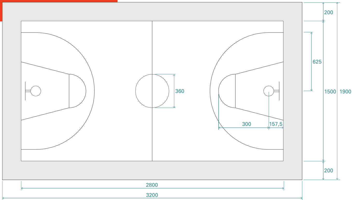
Spießfeld für Rollstuhlbasketball, Grundriss
