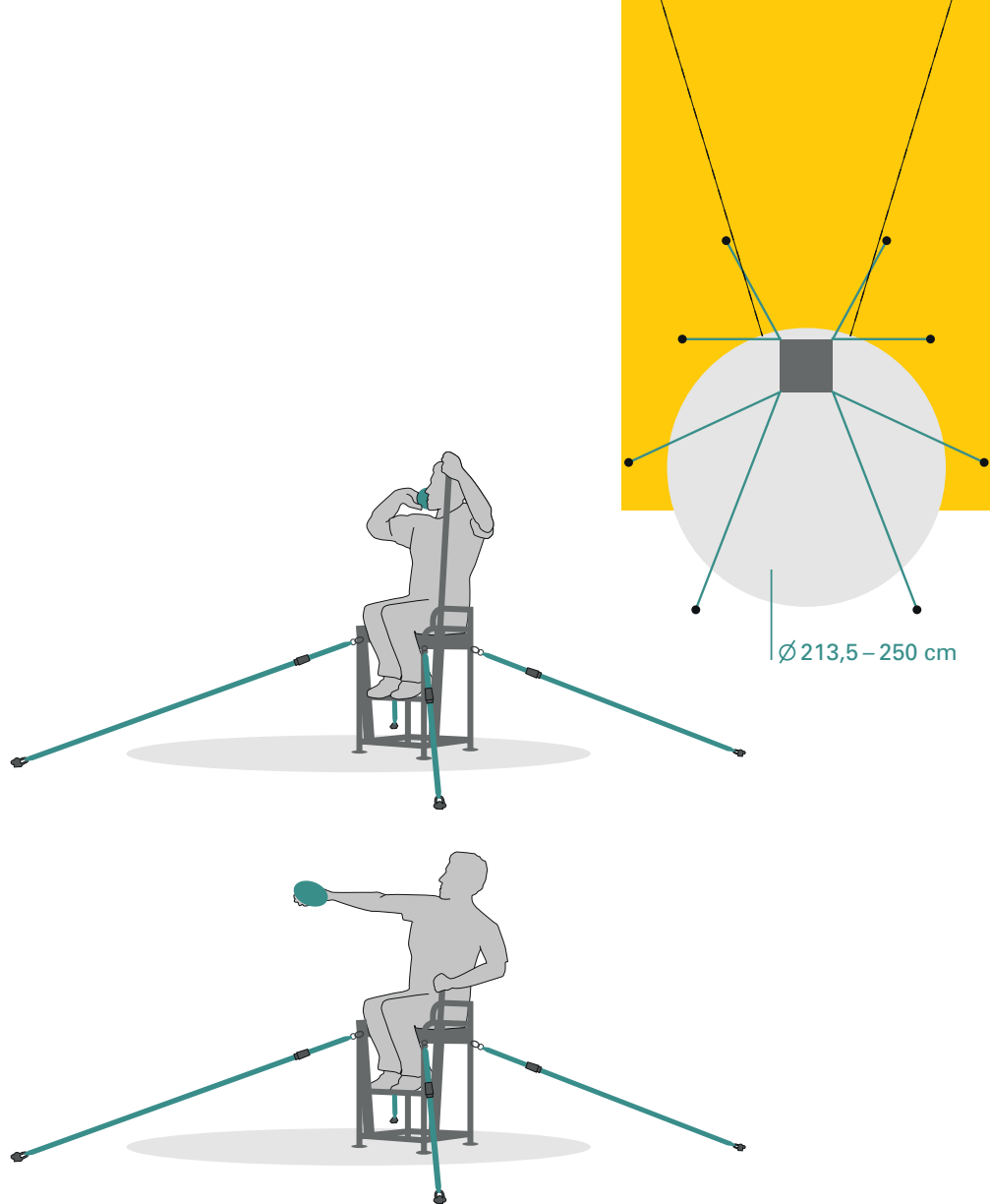
Wurfkreis, Kugelstoßen und Diskuswerfen auf Wurfstuhl, Grundriss, Ansichten
