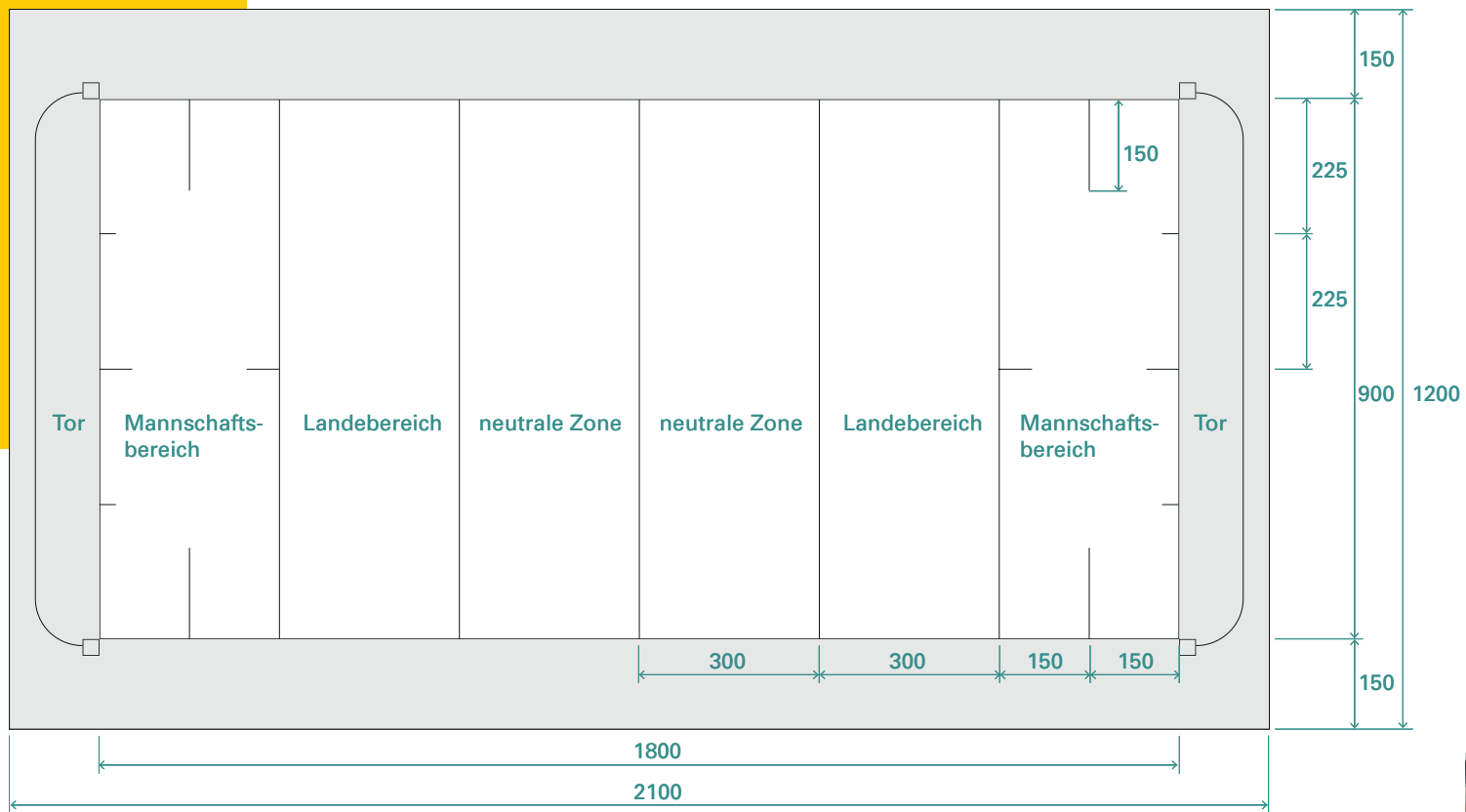
Spielefeld für Goalball, Grundriss
