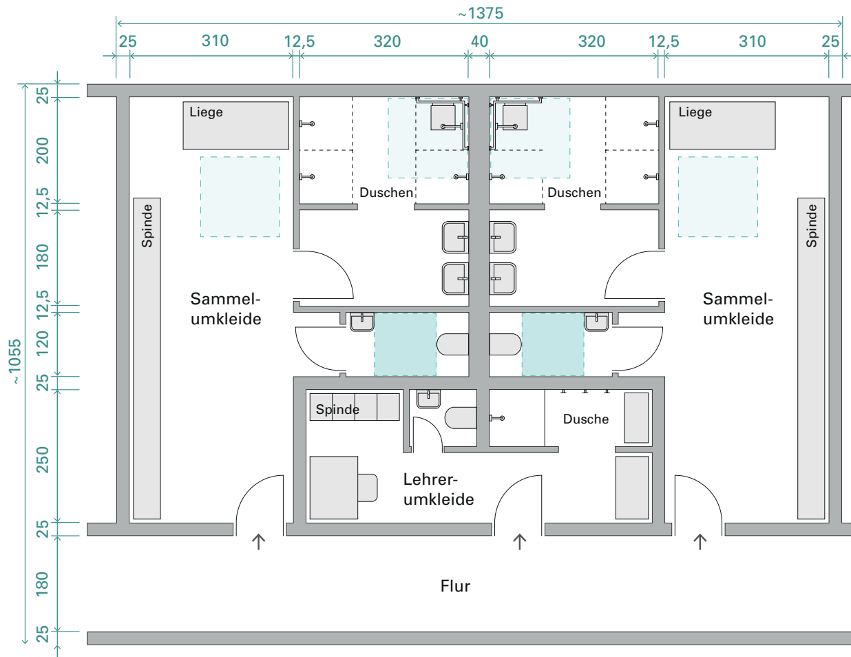
Sammelumkleide mit Waschbereich und WC, Grundriss
